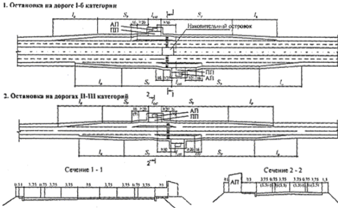
Рис. Б.2. Автобусные остановки на дорогах с пешеходным переходом в одном уровне вне зоны пересечения и примыкания дорог
