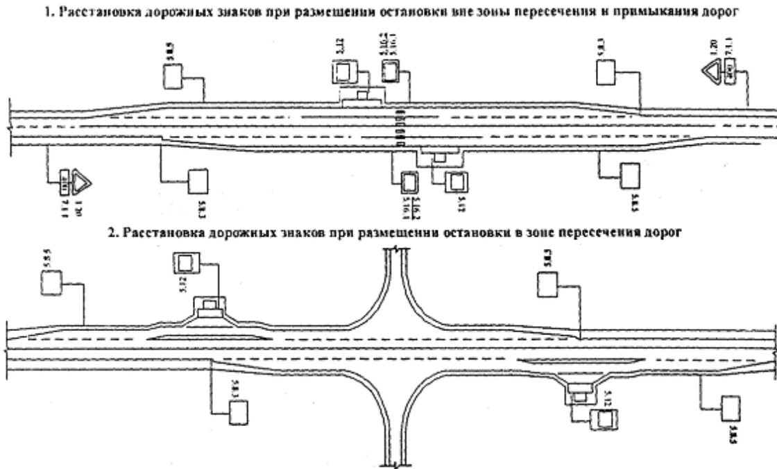
Рис. Б.4. Расстановка дорожных знаков у автобусных остановок
