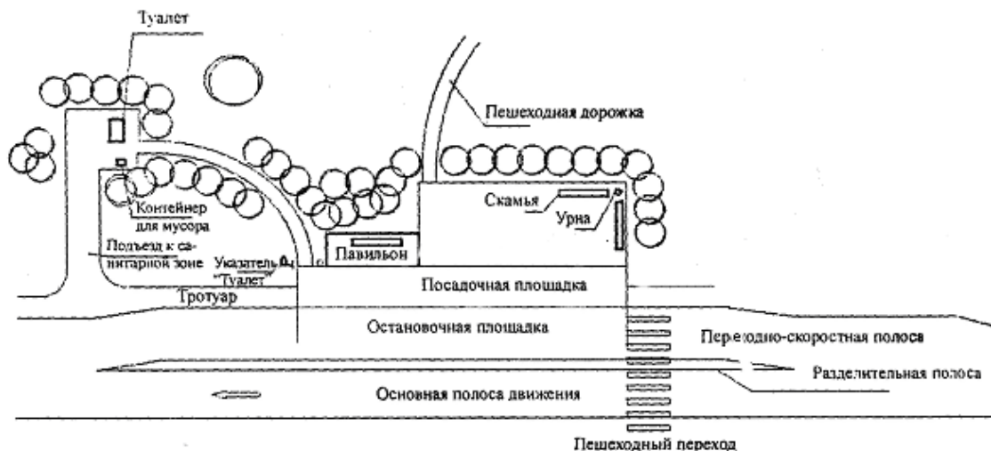
Рис. А.1. Элементы автобусной остановки
